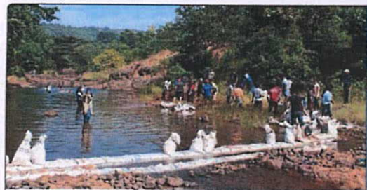
राष्ट्रीय सेवा योजनेच्या माध्यमातून सिंहगड अभियांत्रिकी महाविद्यालयाच्या विद्यार्थ्यांनी वेल्हे तालुक्यातील तोरणा किल्ल्याजवळील टोराणा येथील वनराई बंधाराचे बांधणीचे काम सुरू केले आहे.
